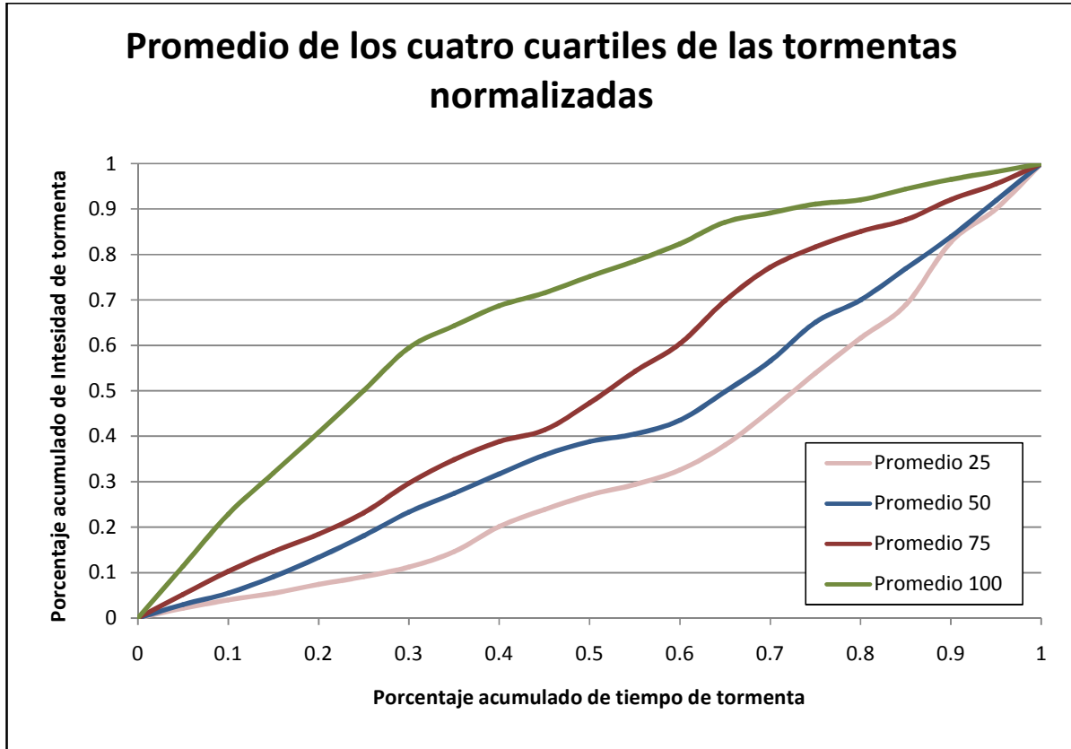
Gráfico No. 14 Promedio de las tormentas normalizadas de los percentiles 25, 50, 75 y 100.
