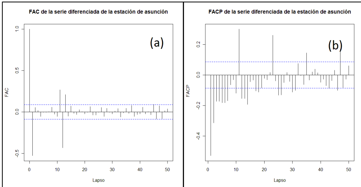
Gráfico No. 2 FAC y FACP de la serie de precipitación diferenciada de la estación de Asunción.
