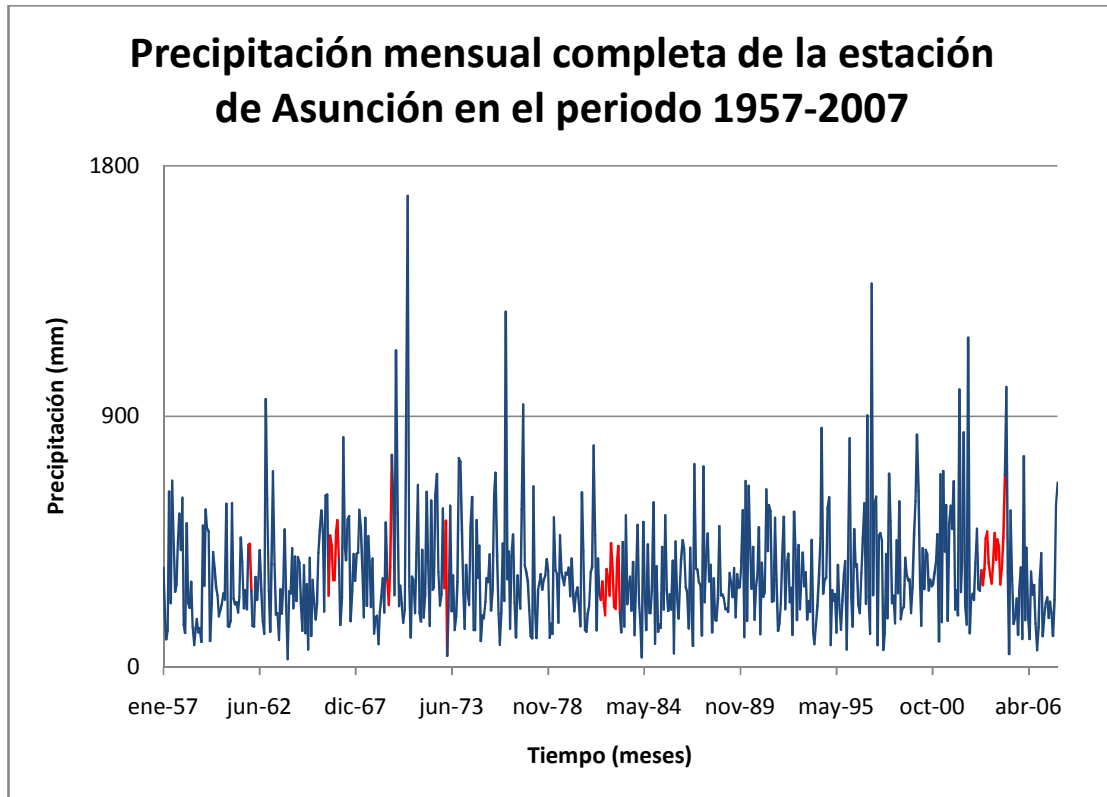
Gráfico No. 3 Serie de precipitación mensual completa de la estación de Asunción en el periodo 1957-2007.
