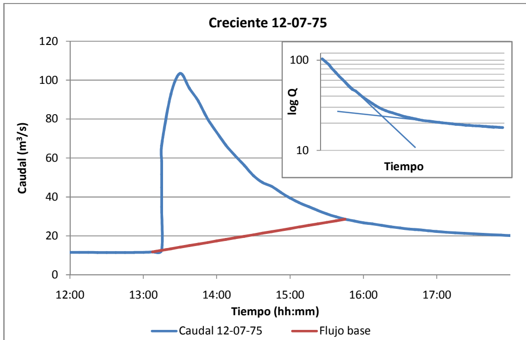
Gráfico No. 19 Ejemplo de Separación de Flujo Base
