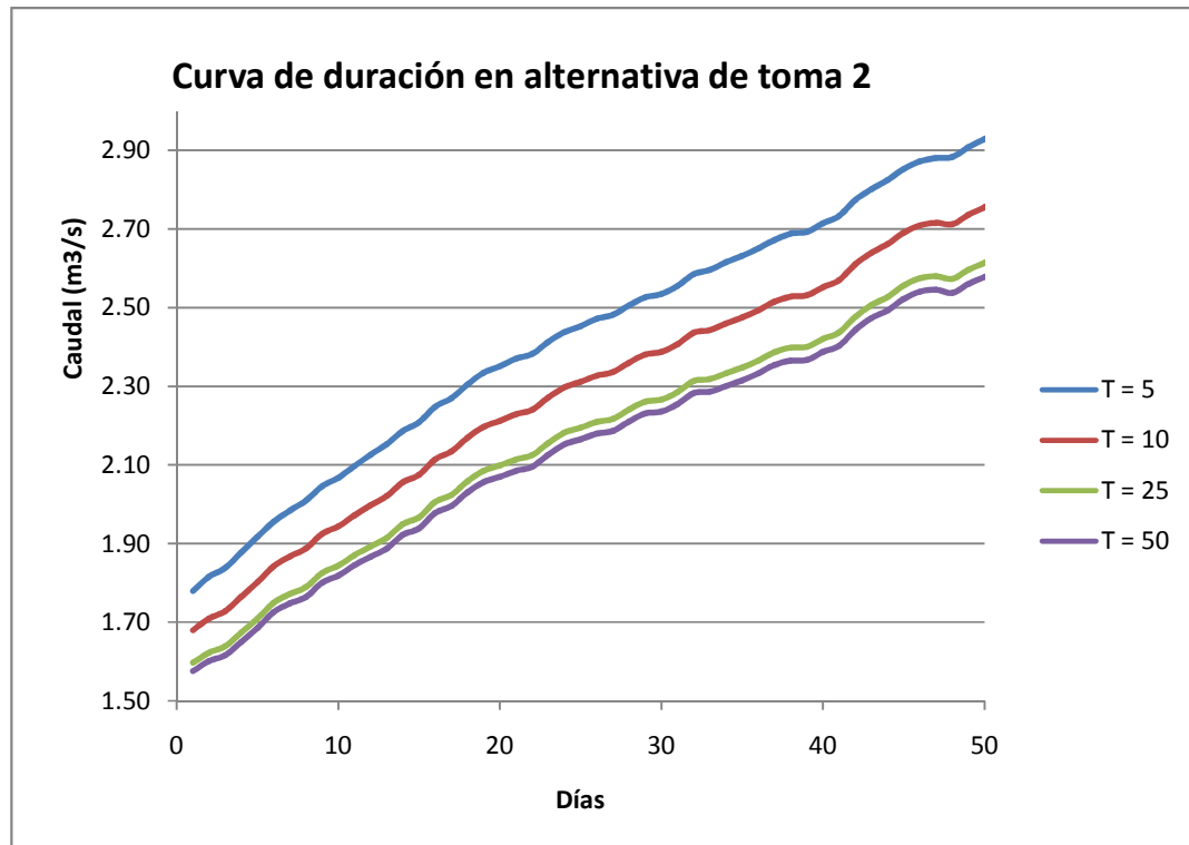
Gráfico No. 10 Curvas de duración para la alternativa No. 2
