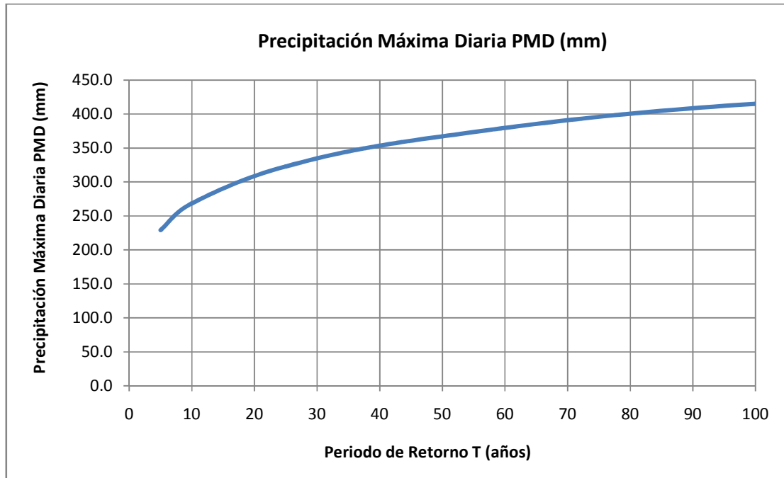
Gráfico No. 18 Precipitación Máxima Diaria para distintos periodos de retorno
