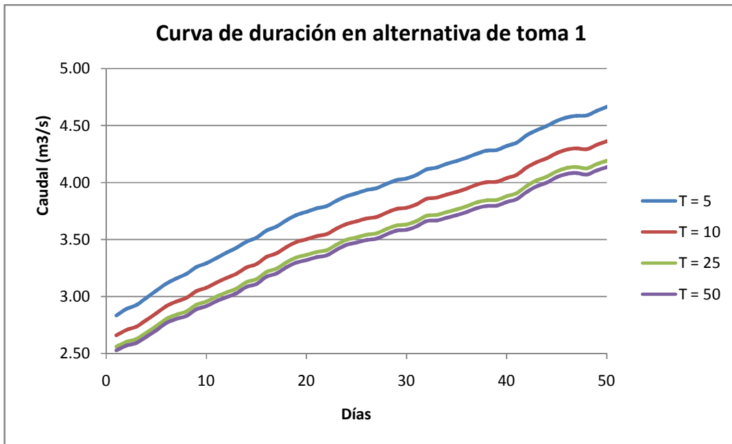
Gráfico No. 9 Curvas de duración para la alternativa No. 1
