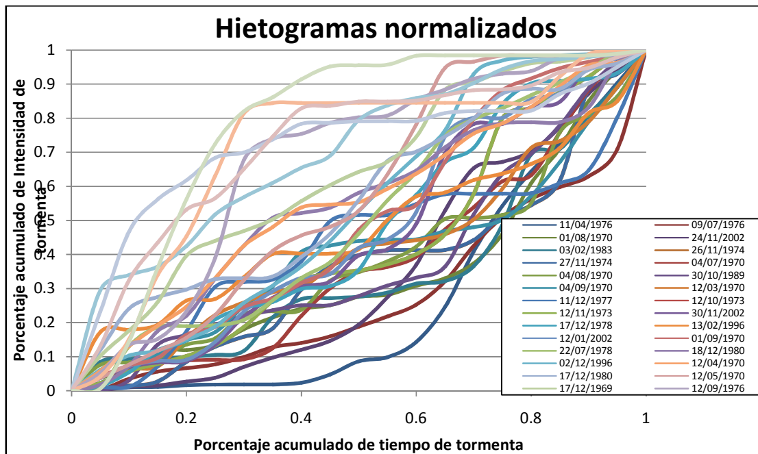
Gráfico No. 13 Tormentas analizadas del registro histórico de la estación pluviográfica de Asunción.
