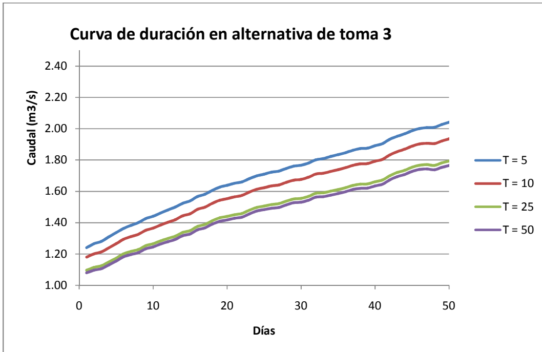
Gráfico No. 11 Curvas de duración para la alternativa No. 3
