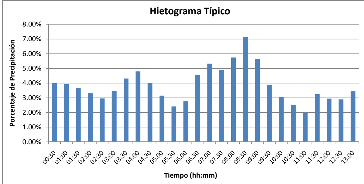
Gráfico No. 15 Hietograma de tormenta típico para la estación de Asunción sobre la cuenca del río Banano.
