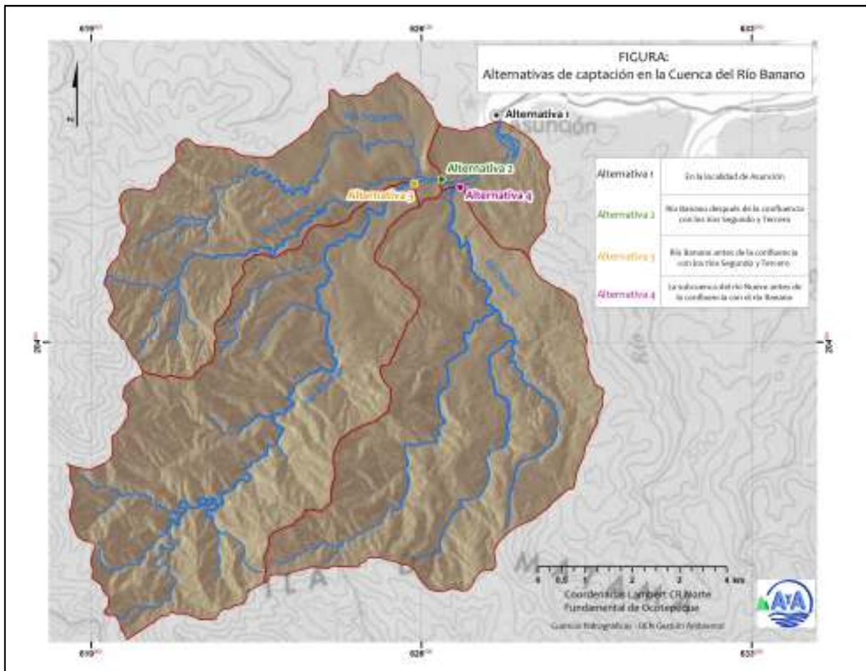
Figura No. 2 Alternativas para la colocación de la toma sobre el río Banano.
