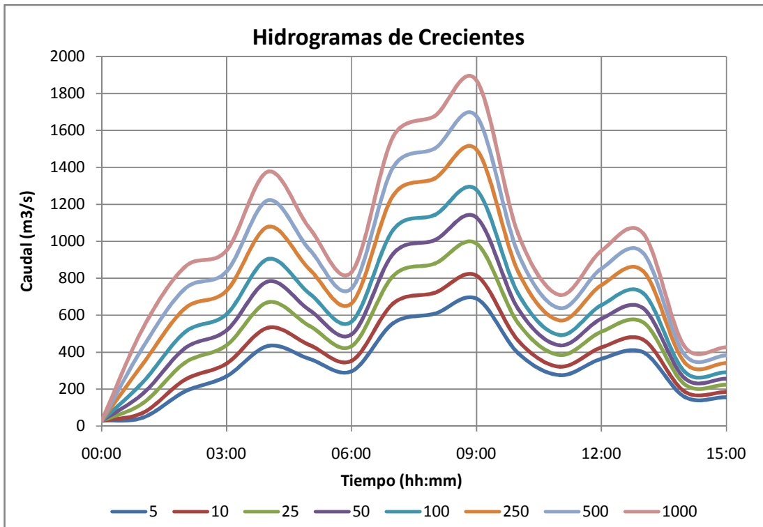
Gráfico No. 21 Hidrogramas de crecientes para diferentes periodos de retorno en la cuenca del río Banano, en la estación de Asunción.
