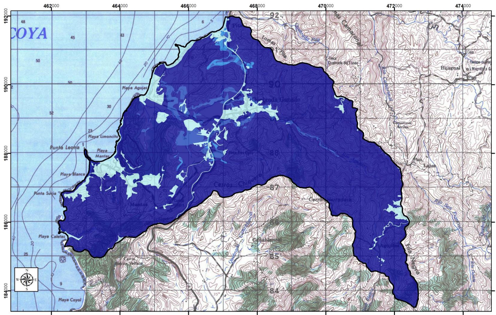
Mapa de Precipitación que infiltra para el mes de noviembre Elaboración: Geól. Christian Corrales Díaz 2017
