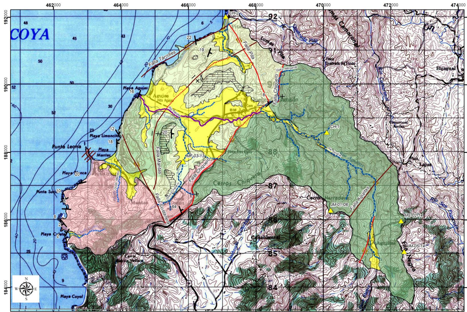
Mapa geológico Elaboración: Geól. Christian Corrales Díaz 2017
