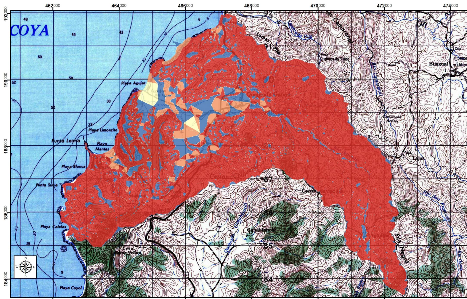
Mapa de Coeficiente de pendiente Kp Elaboración: Geól. Christian Corrales Díaz 2017
